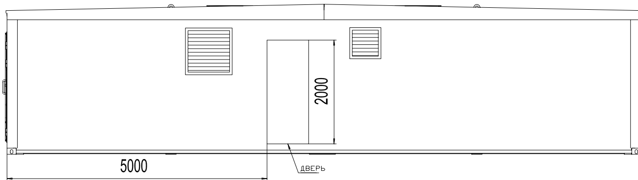
ВИД А
